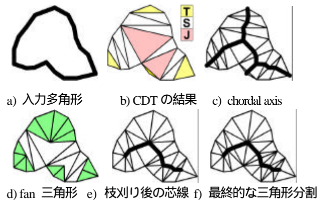
図 13: 芯線の構成
